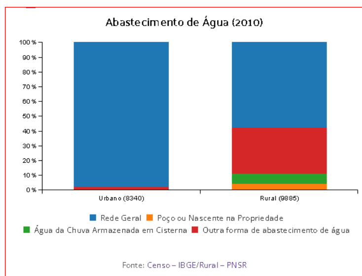
Figura 2 - Abastecimento de Água segundo o Plano Nacional de Saneamento Rural
